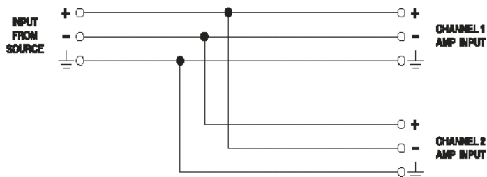
рисунок 2.10 Пользовательский кабель Y-Input
