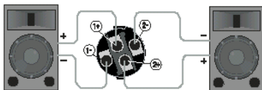
рисунок 2.8. Стерео разводка способ 1: Подключите два динамика к верхнему разъему Speakon
