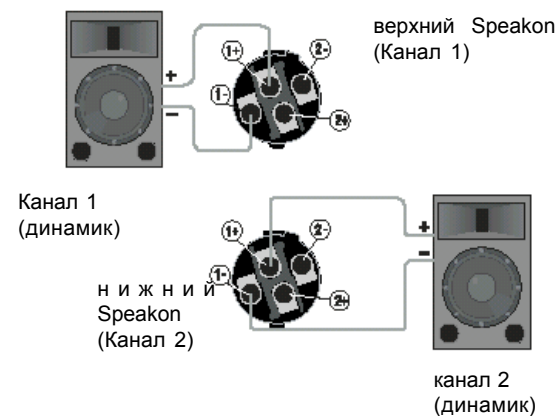
Рисунок 2.9. Стерео разводка, способ 2: Подключите каждый динамик к различным разъемам Speakon
