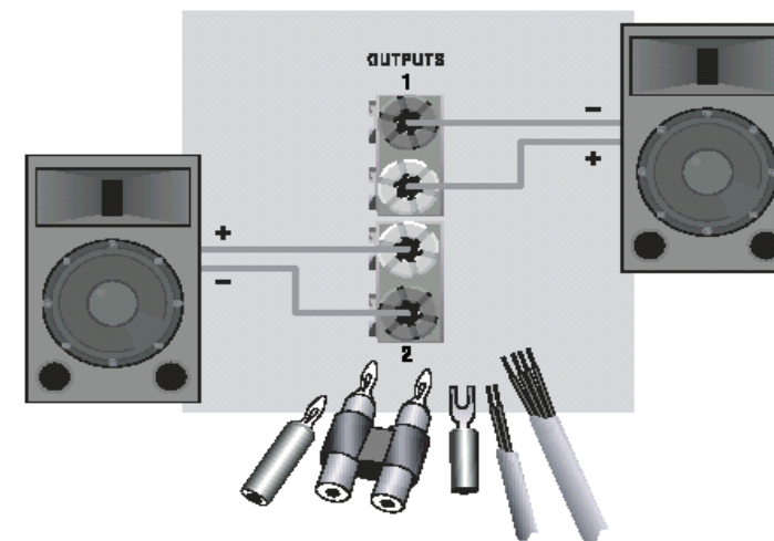
Рисунок 2.6 5-ти полосная винтовая клемма
