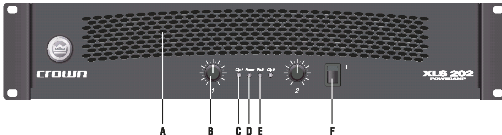
Рисунок 4. 1 Индикаторы и регуляторы передней панели.
