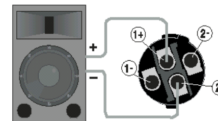
рисунок 2.12 Альтернативная Мостовая - моно разводка: Динамики разведены на верхний разъем Speakon усилителя
