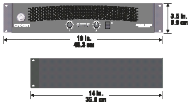
Рисунок 2.1 Размеры
