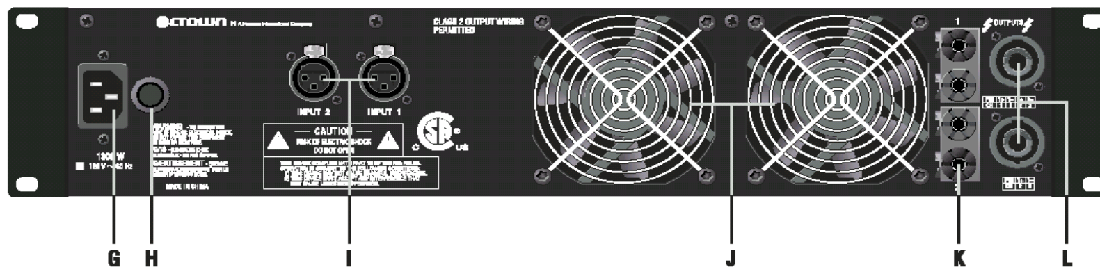
рисунок 4.1 Разъемы и регуляторы тыльной панели
