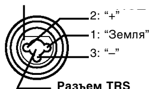
Разъем XLR
