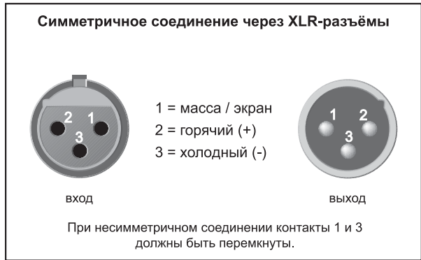
Рисунок 4.3: XLR-соединения
