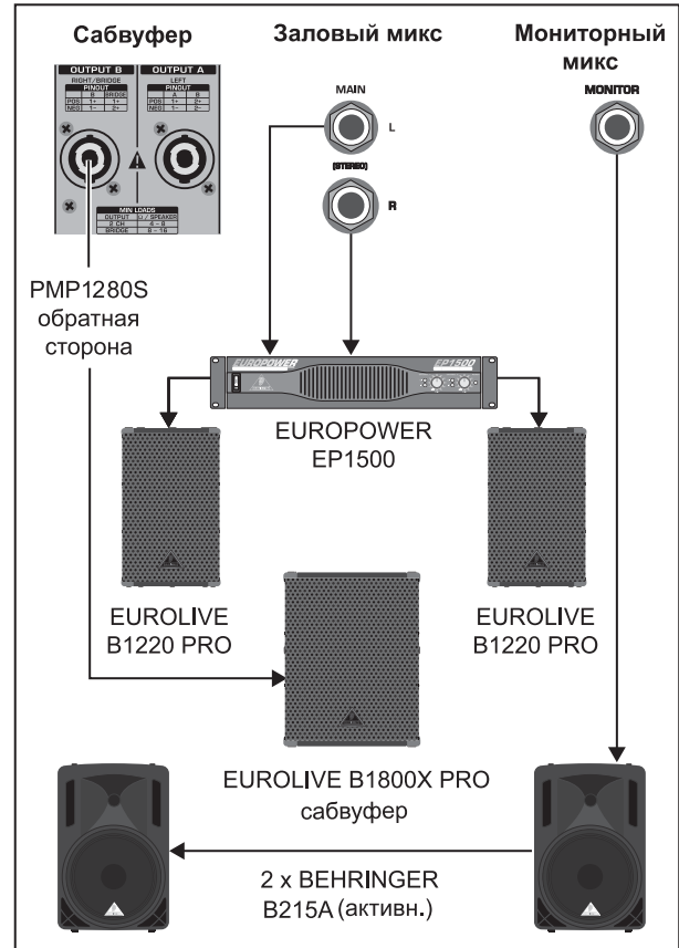
Рисунок 5.4: Работа в одномостовом режиме
