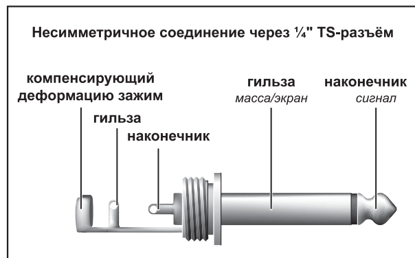
Рисунок 4.1: 6,3-мм-моноштекер
