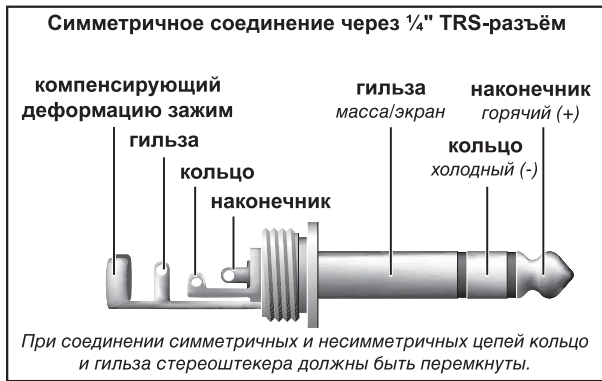
Рисунок 4.2: 6,3-мм-стереоштекер
