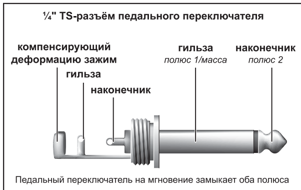
Рисунок 4.4: Моноштекер для педали
