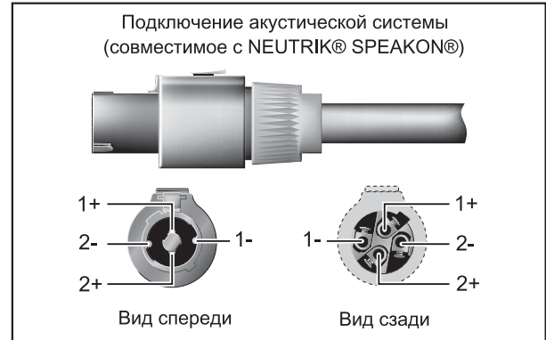
Рисунок 4.6: Профессиональное подключение акустических систем
